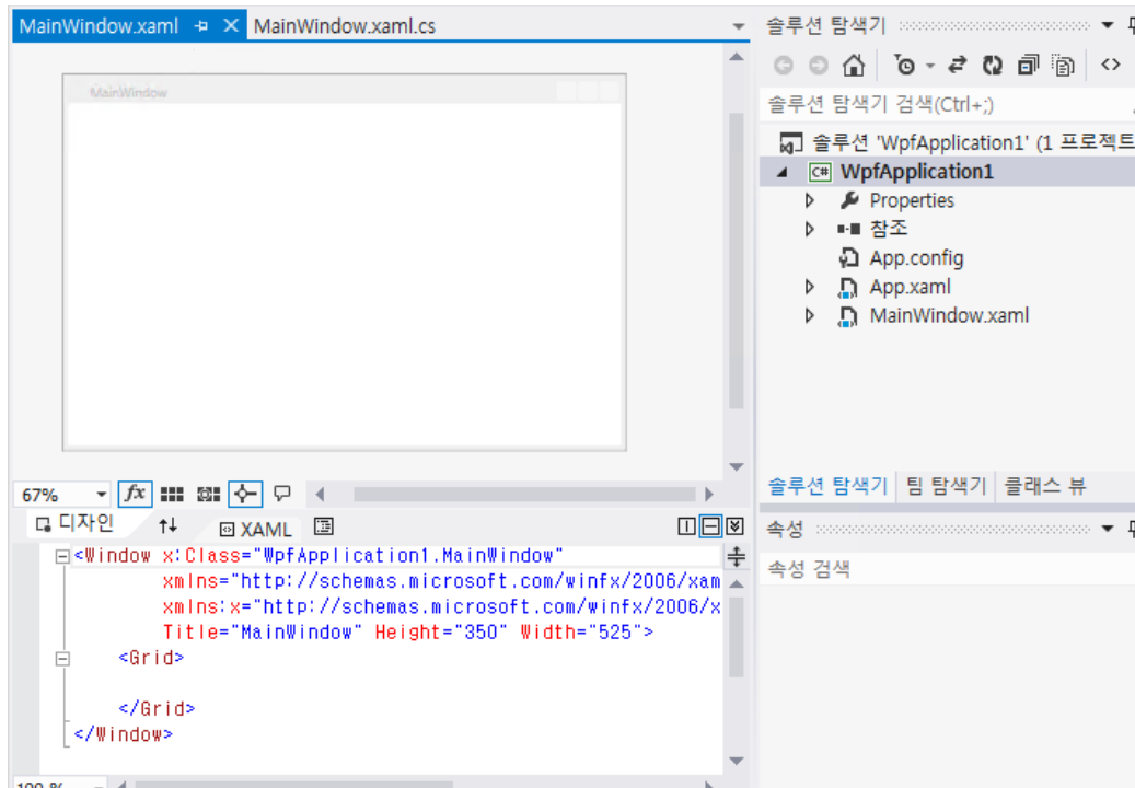
그림 19.37 WPF 프로젝트
