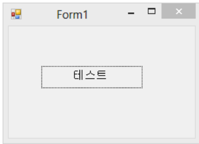
그림 19.29 DottedBoxLabel의 모습
