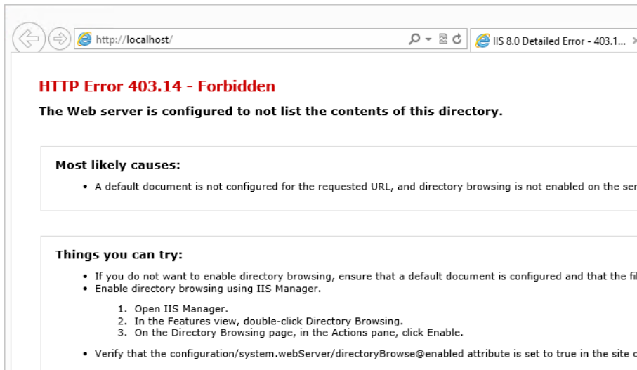
그림 19.72 HTTP 403.14 오류
