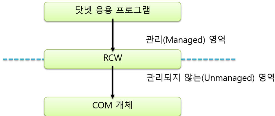
그림 20.12 RCW의 구조
