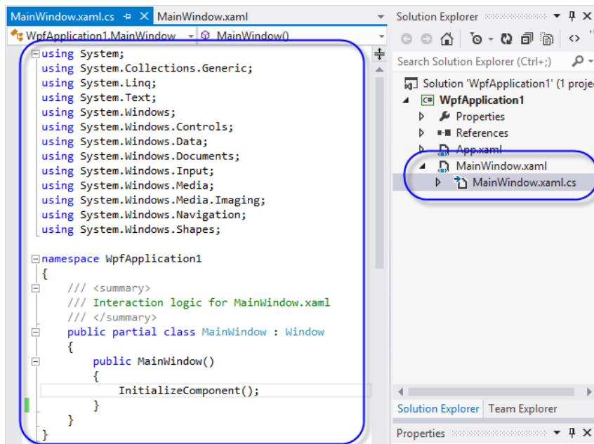
그림 19.38 MainWindow.xaml.cs 파일
